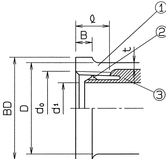
呼び: 2 1/2 ~ 4の端部形状
