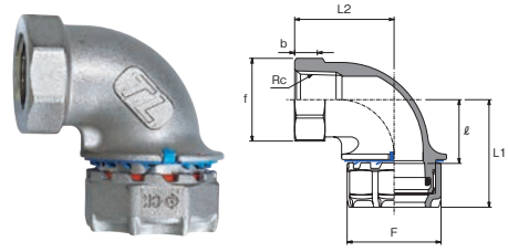
めすアダプターエルボ (AQL)
