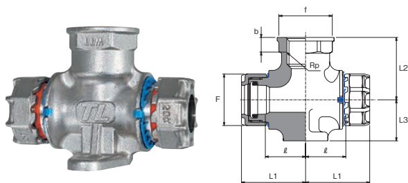
給水栓用座付チース (WTT)
