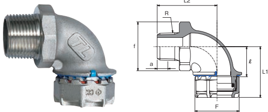
おすアダプターエルボ (APL)
