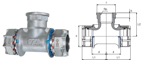
給水栓用チース (WT)
