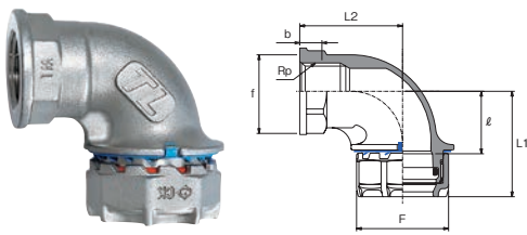
給水栓用エルボ (WL)
