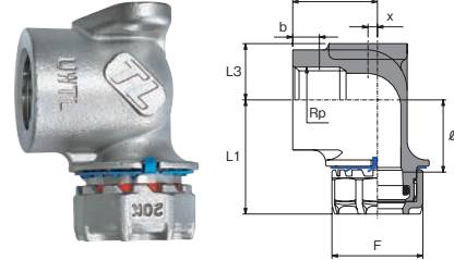
上取型給水栓用座付エルボ (UWTL)
