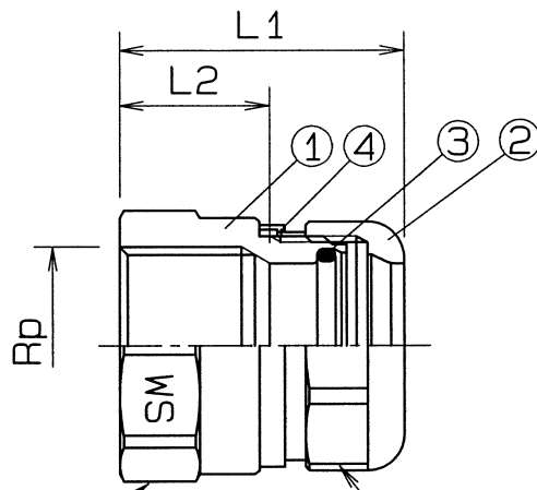
B: 本体の八角二面幅 A: ナットの八角二面幅
